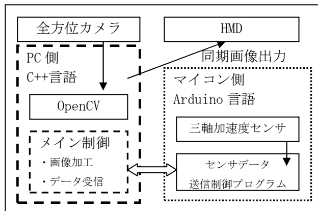
図2 簡略ブロック図
